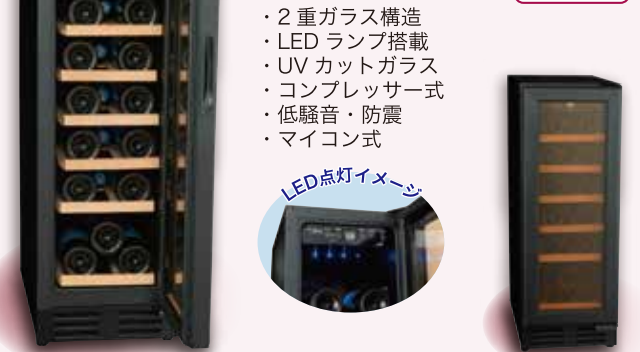
外形寸法：295 × 575 × 820mm (幅 × 奥行 × 高さ)
